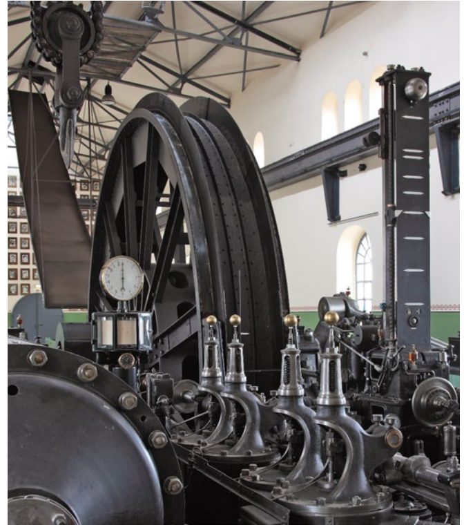
Dampffördermaschine der Zeche Hannover.
